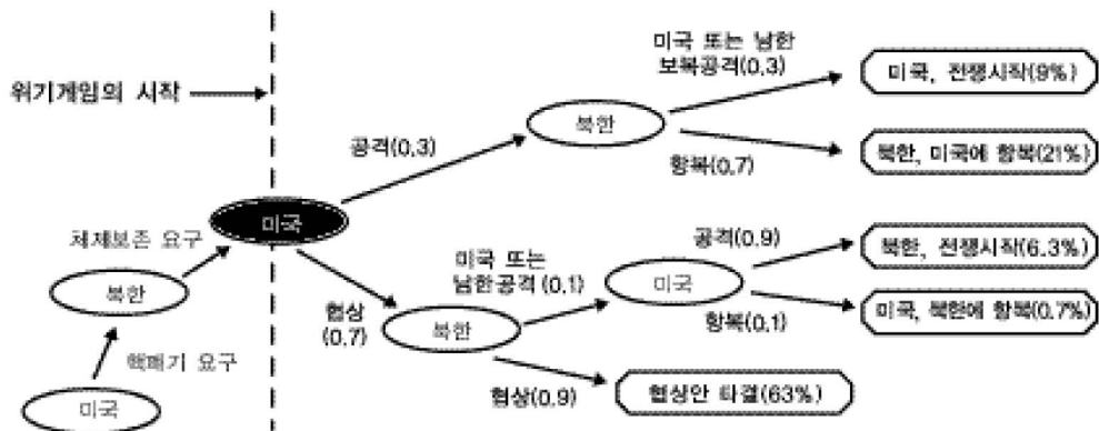
<그림 9> 확률로 보는 결과 가능성
