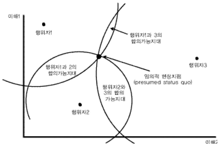
〈그림 5〉 3인 행위자의 윈셋(Win Set) 모형
