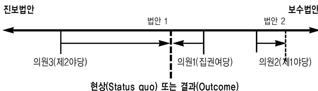
<그림 2> 국회의원 3인의 선호도, 전략에 따른 법안의 결과
