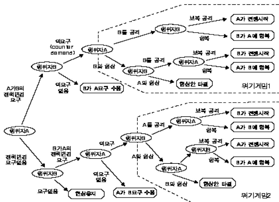
〈그림 7〉 전개형 게임이론 모형
