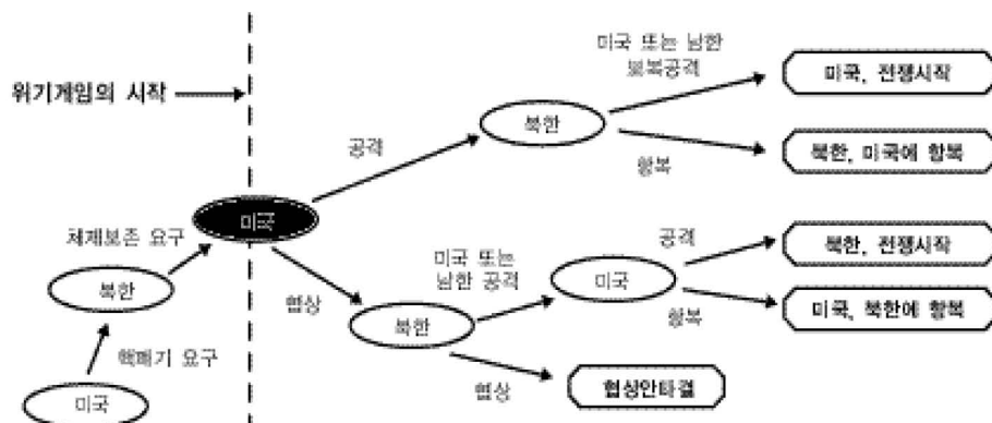
〈그림 8〉 북-미간 핵협상 게임
